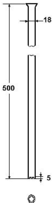
Рисунок 3 - Трубка, вставляемая в пробирку
